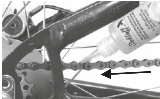
Obr. 159: Mazání řetězu
