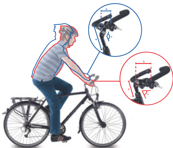
Obr. 114: Poloha u městského (modrá) a trekkingového kola (červená) při změně úhlu
