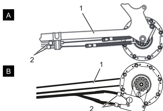
Obr. 191: Nastavovací pouzdra (2) řazení ve dvou alternativních provedeních (A a B) s ovládním dvěma lanky na zadní rámové stavbě (1)
